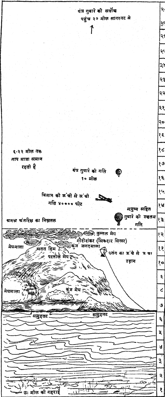
चित्र १५७—समुद्रतल से सार्द्धस मील अन्तरिच तक मनुष्य के कारणों और उपकरणों की पहुँच की सीमा [ टायमसन का अरुकारण ]
